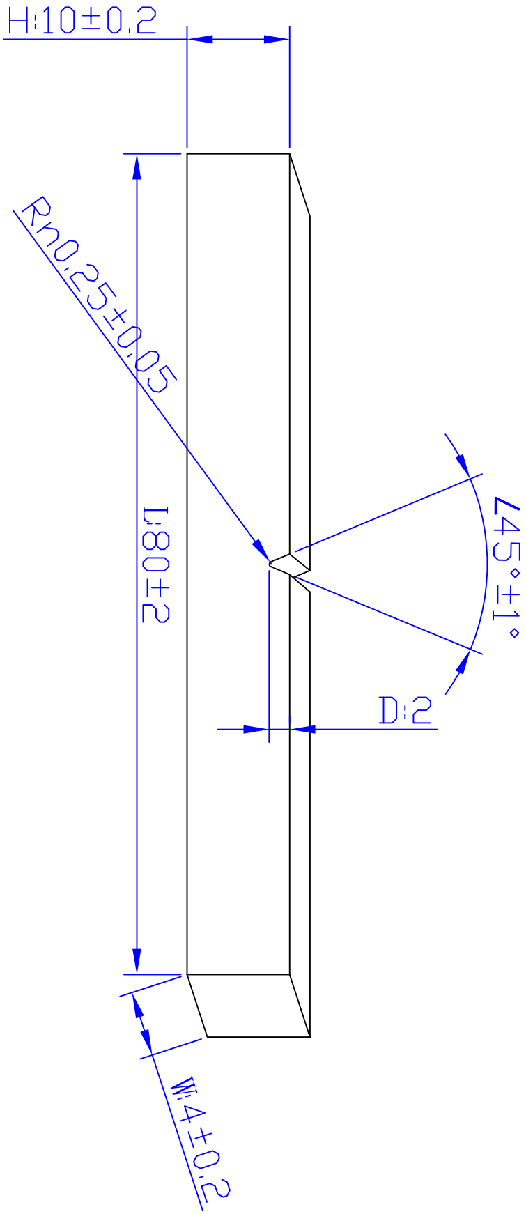
国标冲击样条尺寸(A型)
